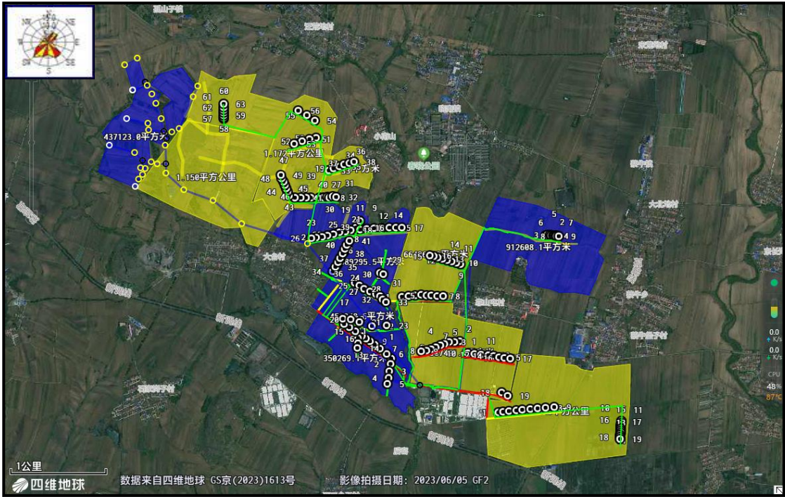
图 6-3 本项目的水肥管网示意图
