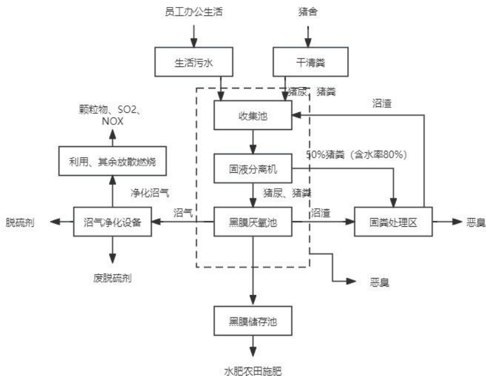
图 6-1 项目污染物处理及综合利用图
