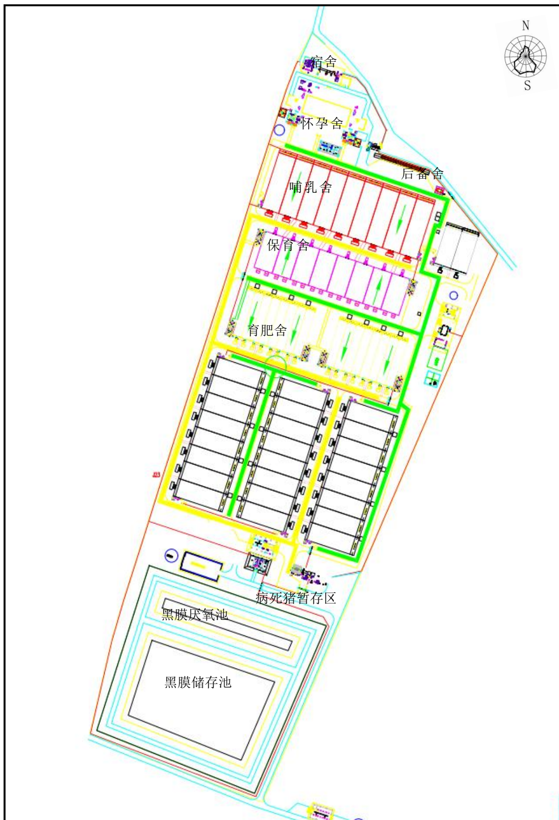
图 3-4 辽宁铁岭牧原农牧有限公司铁岭十一场实际平面布置图
