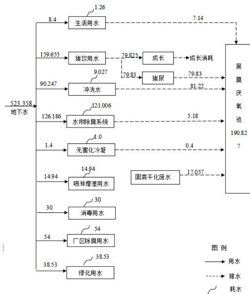
图 3-4 项目实际水量平衡图 单位：m 3 /d
