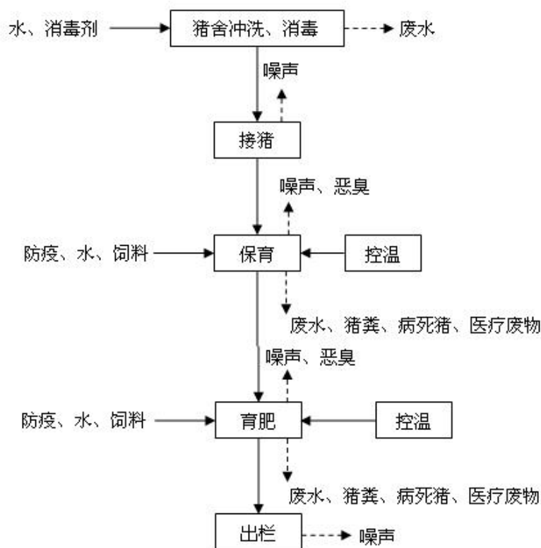
图 2.2-2 养殖过程及产污环节图
