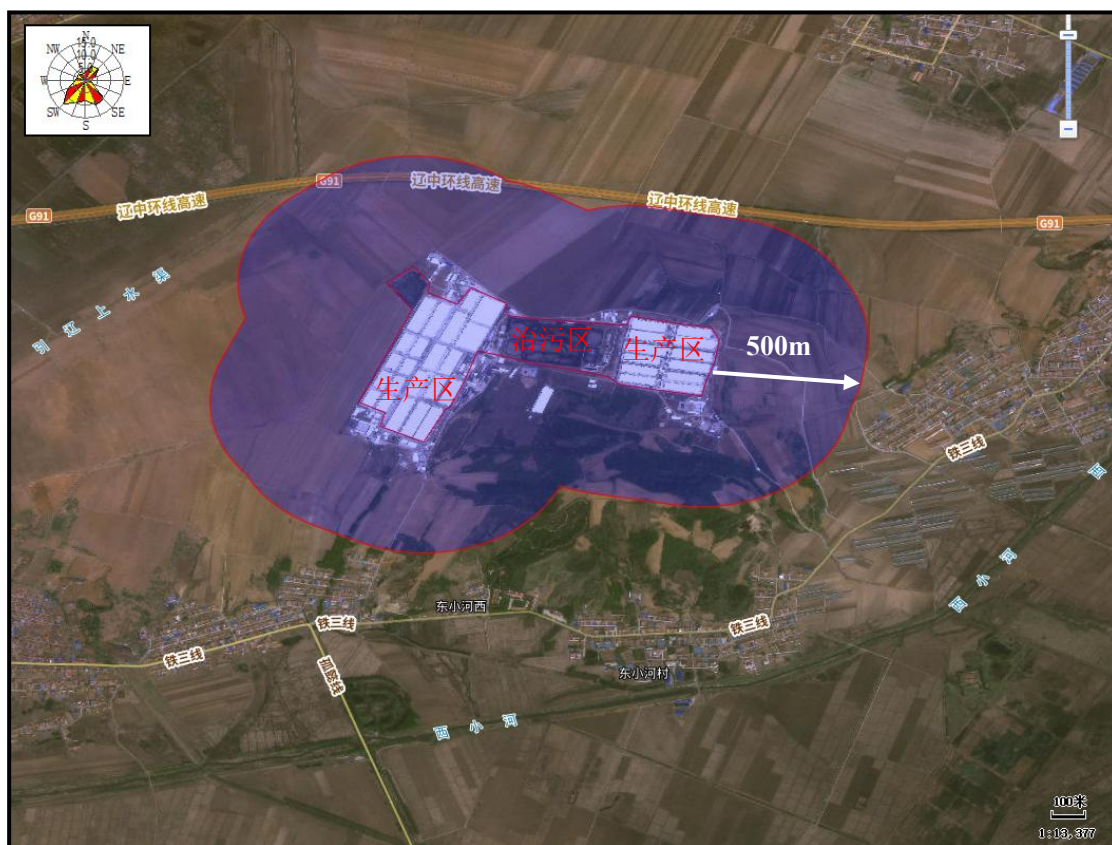
图 7-1 项目现状卫生防护距离包络线图
