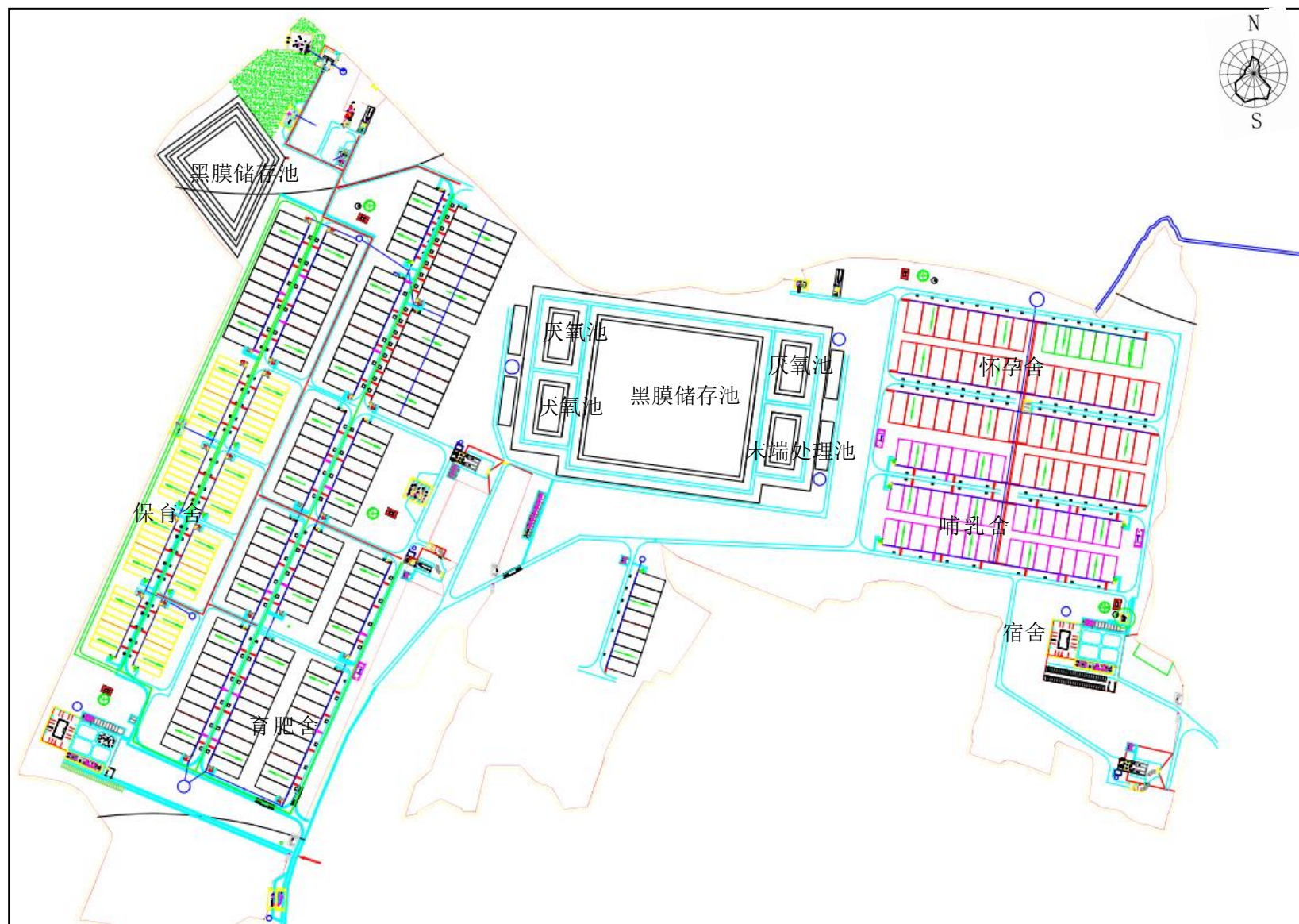
图 3-4 辽宁铁岭牧原农牧有限公司铁岭二场实际平面布置图
