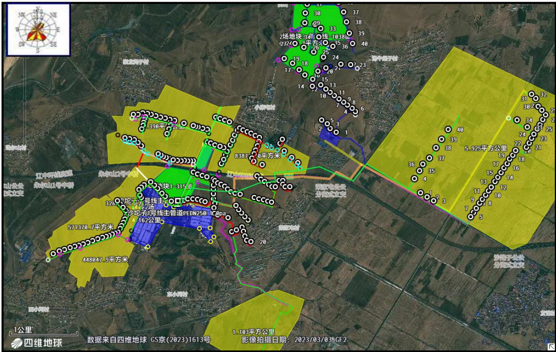
图 6-3 本项目的水肥管网布置示意图
