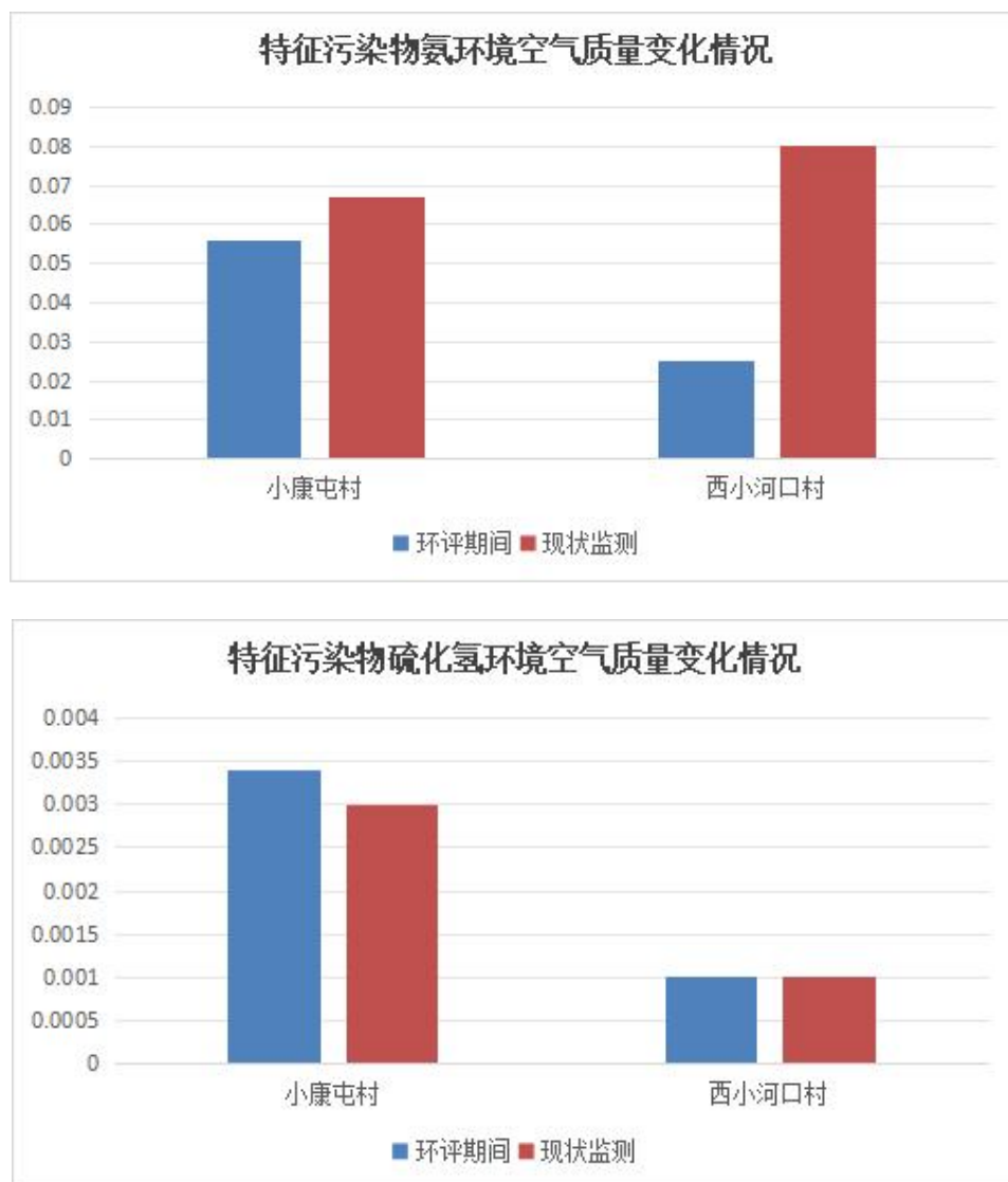
图 5-2 特征污染物环境空气质量变化情况
