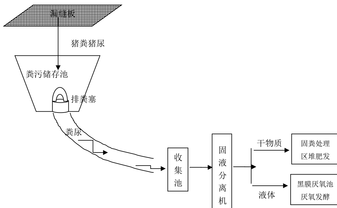
图 4-3 项目清粪工艺示意图
