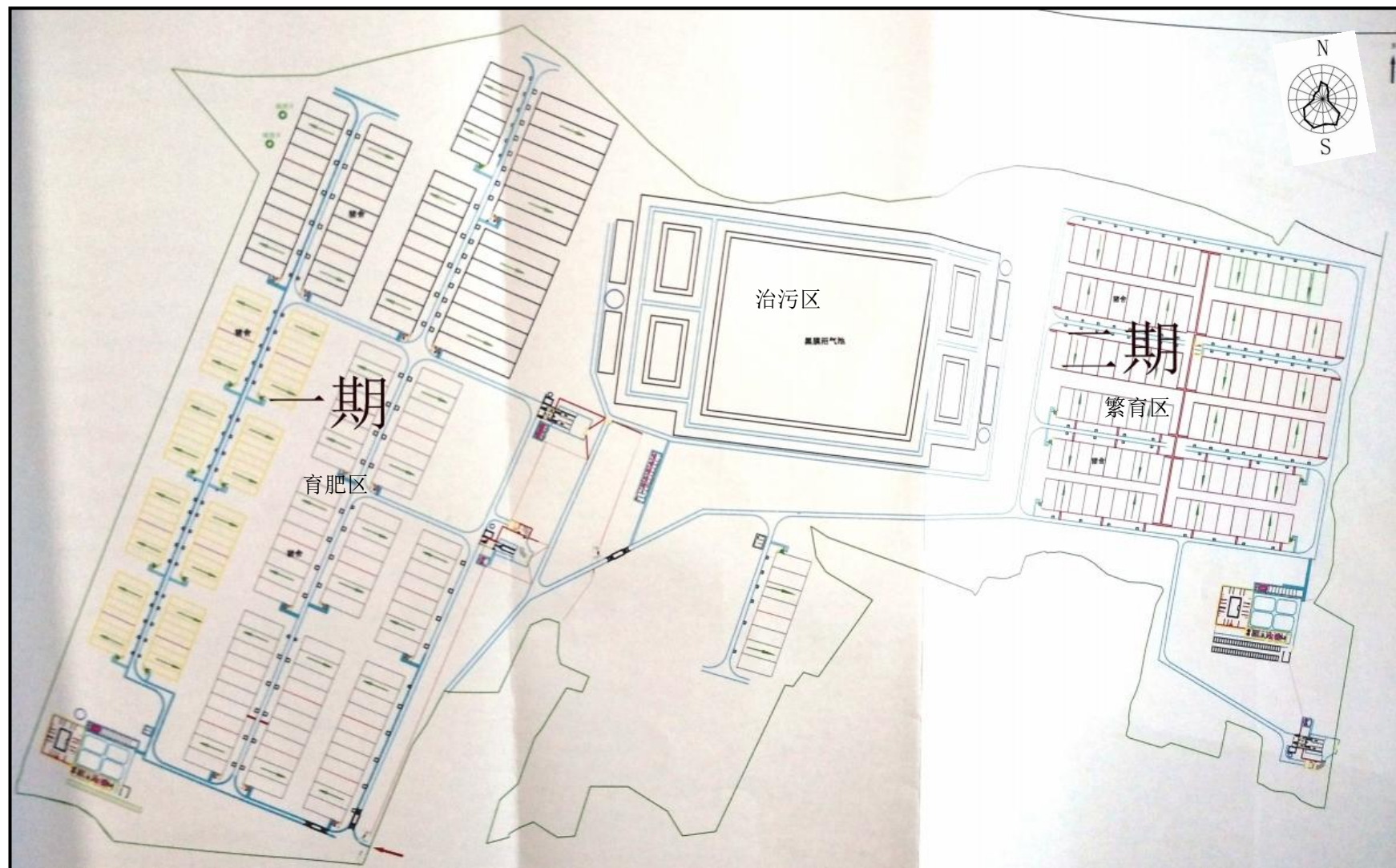
图 3-3 辽宁铁岭牧原农牧有限公司铁岭二场设计厂区布置图
