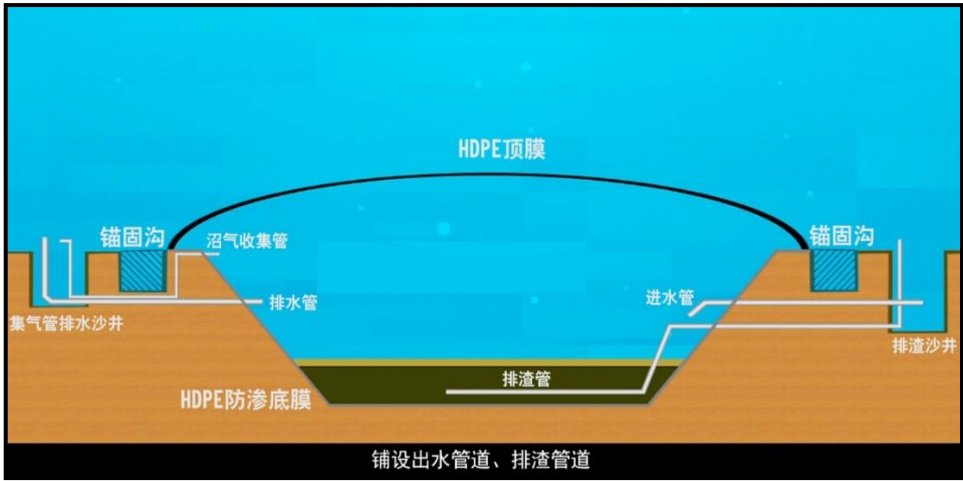
图 6-2 盖泻湖（黑膜）沼气池结构示意图
